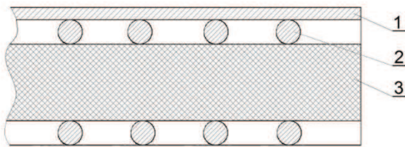
Rys. 2. Schematyczny przekrój uproszczonego modelu sztucznego dna szybu [3].
