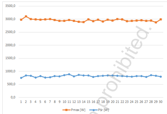
Rys. 6. Porównanie wartości P_{max} oraz P_{sr} pobieranej przez rozrusznik podczas rozruchu
