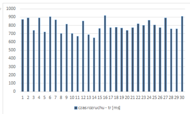
Rys. 8. Wartości czasu rozruchu w podziale na próbki
