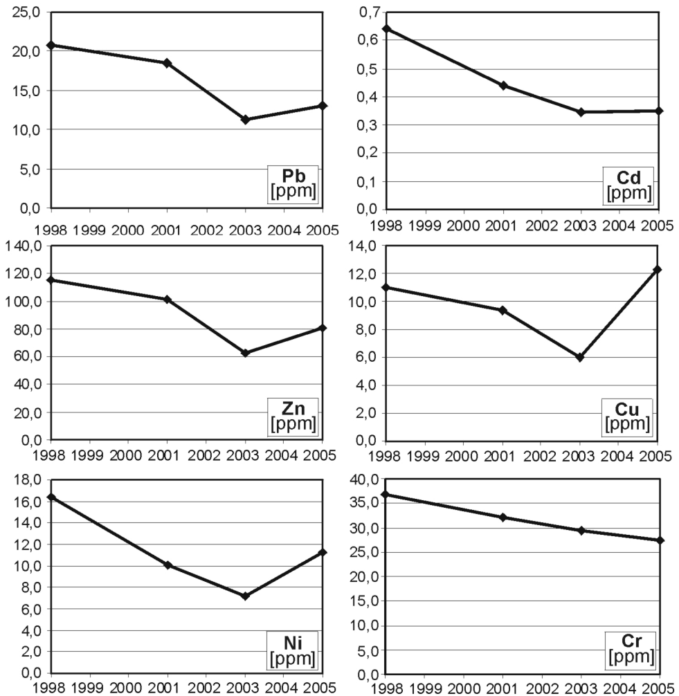
Rys. 2. Wartości średnie zanieczyszczenia osadu zbiornika w Zesławicach w latach 1998-2005
