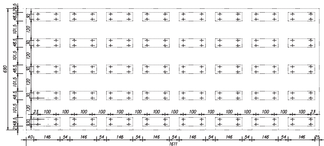
Rys. 1. Rzut powierzchni stendu przed modernizacją
