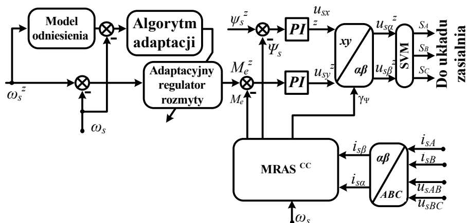
Rys. 1. Schemat blokowy bezczujnikowego układu bezpośredniego sterowania momentem – DTC
