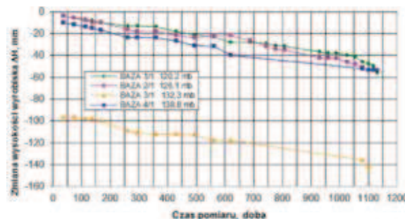
Rys. 10. Zmiana wysokości chodnika nadścianowego 2-Z1, Z2
