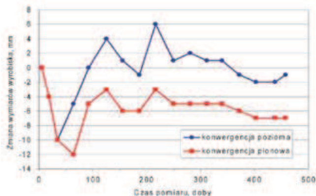
Rys. 13. Zmiana wymiarów chodnika pośredniego E1 Fig. 13. Change in the dimensions of sub-drift E1
