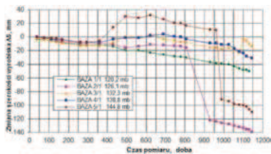
Rys. 9. Zmiana szerokości chodnika nadścianowego 2-Z1, Z2
