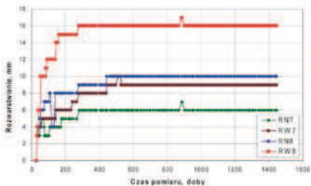
Rys. 14. Rozwarstwienia w stropie chodnika pośredniego E1 Fig. 14. Stratification in the roof of sub-drift E1
