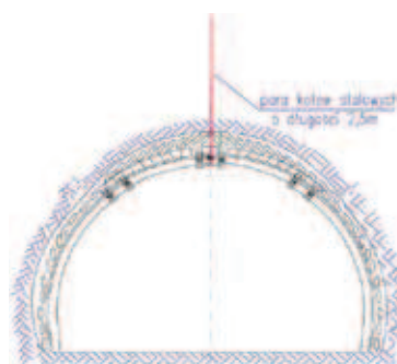
Rys. 5. Schemat obudowy w pochylni zachodniej pokład 358/1 Fig. 5. Scheme of housing in the west inclined drift, seam 358/1
