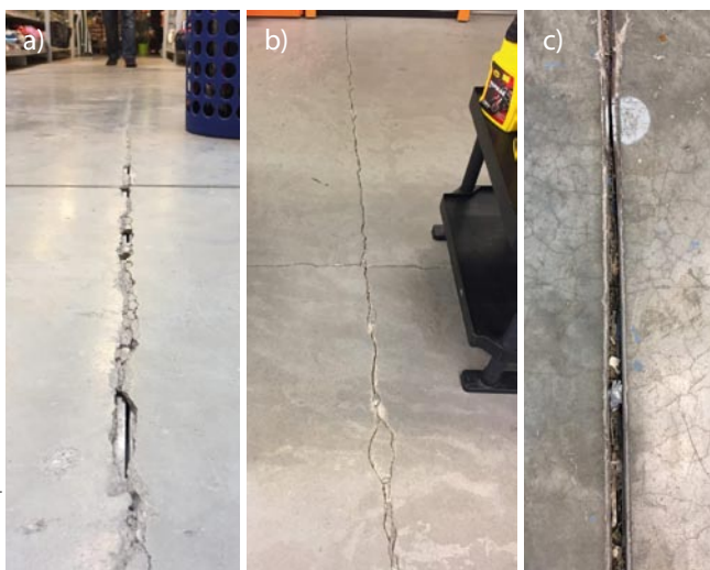
Rys. 9. Uszkodzenie posadzki i dylatacji konstrukcyjnej w wyniku błędów: a) wykonawczych, b) projektowych – brak nacięć, c) eksploatacyjnych – brak zabezpieczenia przed zamuleniem
