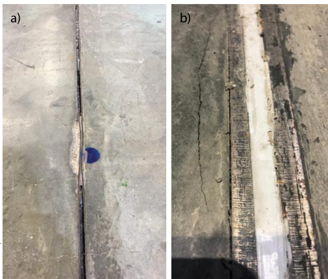
Rys. 8. Uszkodzenie eksploatacyjne krawędzi posadzki przy dylatacji konstrukcyjnej: a) wygięcie profilu, b) wykruszenie krawędzi i wytarcie płaskowników
