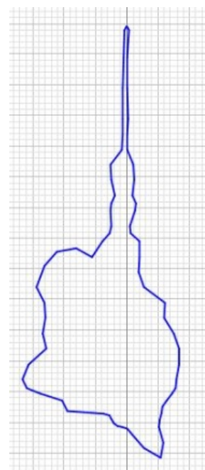
Ryc. 7. Przekrój pionowy kawerny Fig. 7. Vertical section of cavern
