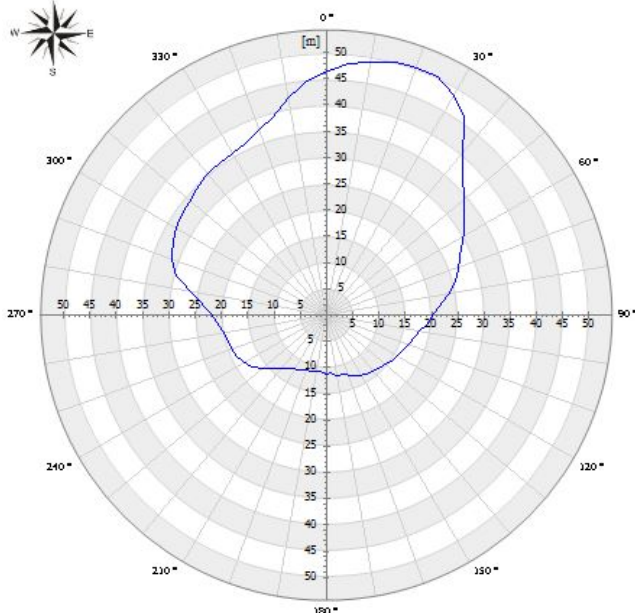
Ryc. 6. Przekrój poziomy kawerny Fig. 6. Horizontal section of cavern
