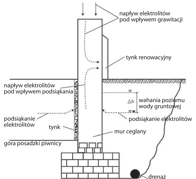
Rys. 1. Przekrój ściany fundamentowej zawilgacanej przez wody gruntowe (opracowanie własne)
