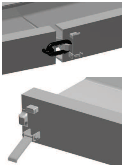
Rys. 1. Szybkozłącze rynien przenośnika z zabezpieczeniem magnetycznym [1]
