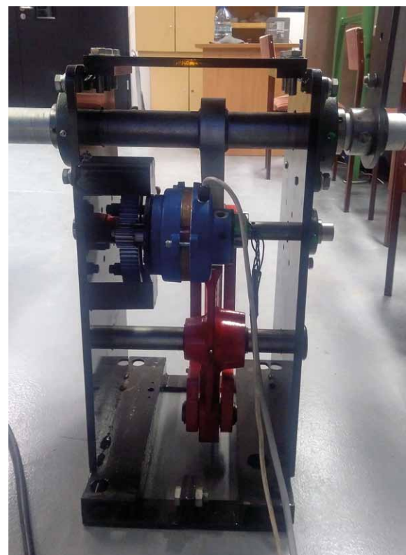
Rys. 6. Napęd rogakowy z opracowanym silnikiem
