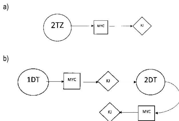
Rys. 14. Schemat obróbki na docierakach: a) docieranie wstępne i wykończeniowe, wymagające wymiany tarcz, b) zastosowanie dwóch docierarek; do obróbki wstępnej i wykończeniowej
