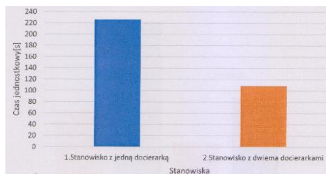
Rys. 15. Porównanie czasów jednostkowych w wariantcie II technologii docierania
