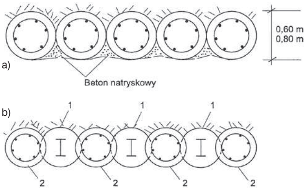
Rys. 7. Schemat palisady [1]: (a) z pali stykających się pobocznicami, (b) z pali wzajemnie wciętych: (1) pale pierwotne, (2) pale wtórne
