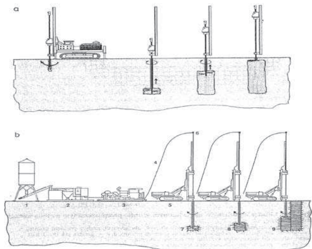
Rys. 8. Iniekcja strumieniowa [2]: a) schemat etapów realizacji, b) zestawu stosowanego sprzętu
