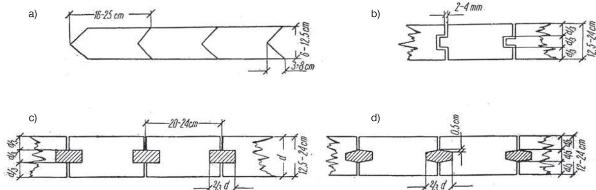
Rys. 1. Łączenie ścian szczelnych drewnianych [3]
