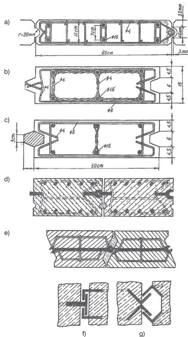
Rys. 3. Przekroje poprzeczne brusów żelbetowych [4]
