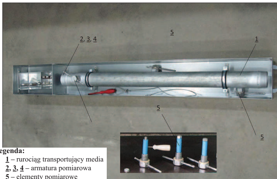
Fot. 1. Elementy stanowiska do monitorowania mikrośrodowiska w instalacjach sanitarnych i technologicznych (Biuletyn Urzędy Patentowej z dnia 10.09.2012 r., nr 19(1010)/2012) fot. Z. Staszewski, 2013r.
