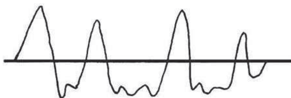
Rys. 1. Schemat powierzchni polimerów – odchylenia spowodowane obrostami mikrobiologicznymi od płaszczyzny odniesienia (nowego rurociągu)
