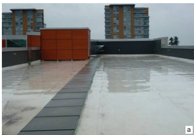
Il. 8. System gospodarki wodą: a) dach obiektu wykonany z białej folii izolacyjnej tworzący rodzaj wanny służącej do zbierania wody deszczowej, b) kanały i rowy, które w naturalny sposób rozprzewadzą oczyszczoną wodę na działce
