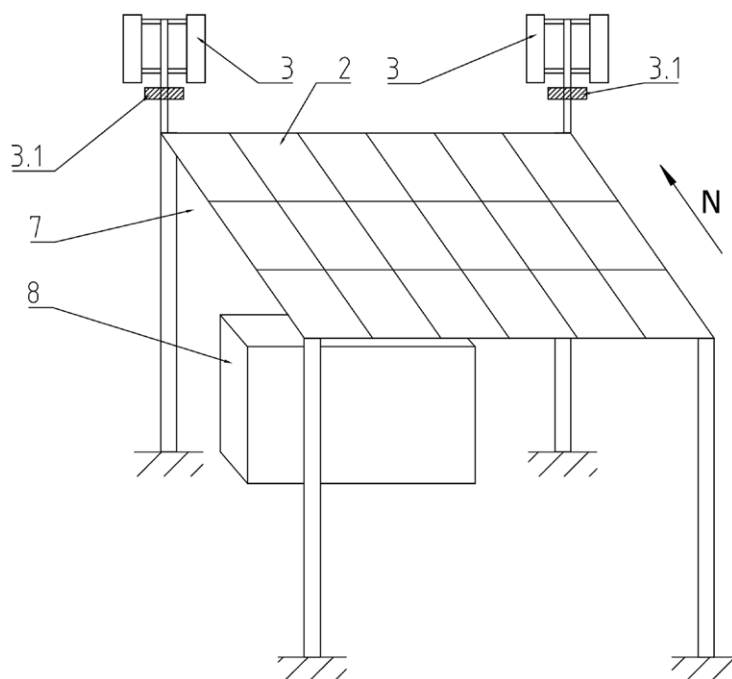
Rys. 3. Wiaty z panelami fotowoltaicznymi i dwiema elektrowniami wiatrowymi [1]
