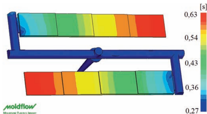
Rys. 3. Położenie frontu strumienia tworzywa w fazie wypełniania gniazda formy schodkowej polipropylem Moplen HP648T z poroforem
