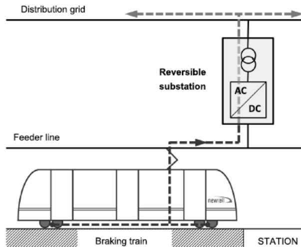
Fig. 12. Schematic of reversible substations in urban rail Rys. 12. Schemat podstacji falownikowej w kolei miejskiej
