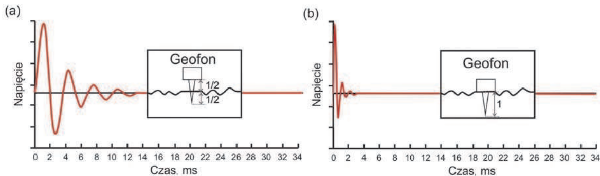
Rys. 9. Odpowiedź napięciowa geofonu niewłaściwie przytwierdzonego do podłoża (a) oraz geofonu prawidłowo przytwierdzonego (b) na podstawie [10]
