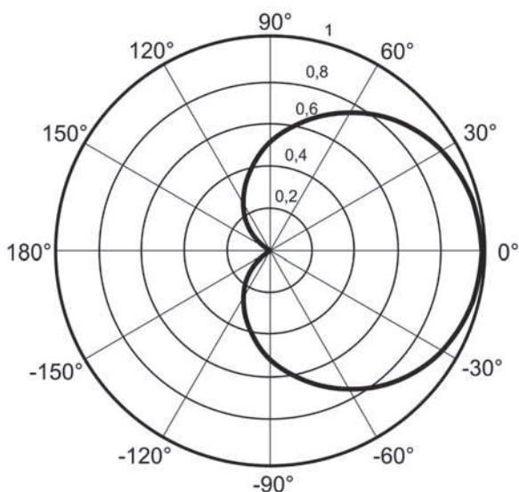
Rys. 10. Przykład charakterystyki kierunkowej geofonu jedno-składowego
