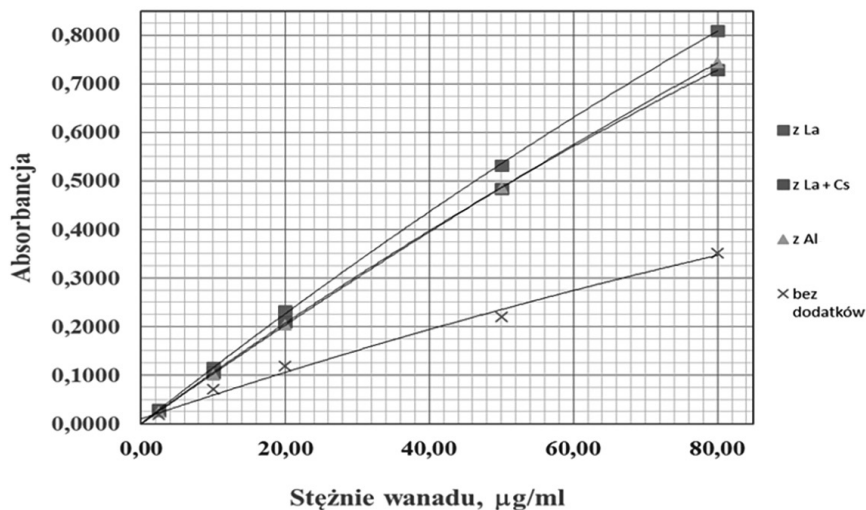
Ryc. 1. Wpływ dodatków: chlorku lantanu (La), chlorku lantanu i ceszu (La + Cs) i glinu (Al) na zależność absorbancji wanadu od stężenia w zakresie stężeń wanadu 2,50 ÷ 80,00 \mu\text{g/ml}
