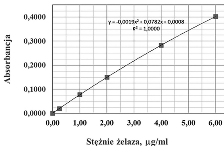
Ryc. 3. Krzywa wzorcowa oznaczania wanadu metodą F-AAS, przy długości fali 318,5 nm, z atomizacją w bogatym płomieniu acetylen-podtlenek azotu
