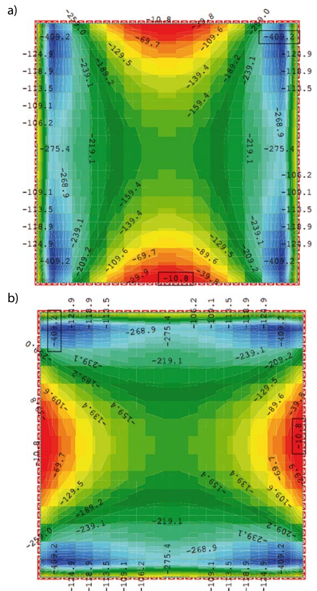
Rys. 9. Mapa sił membranowych a) n_{yy} , b) n_{xx}
