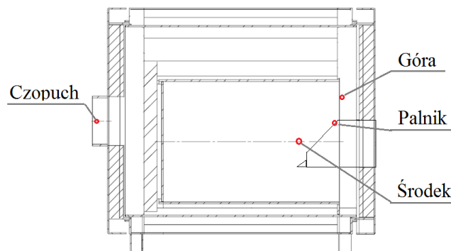
Rys. 7. Rozmieszczenie termopar wewnątrz komory spalania
