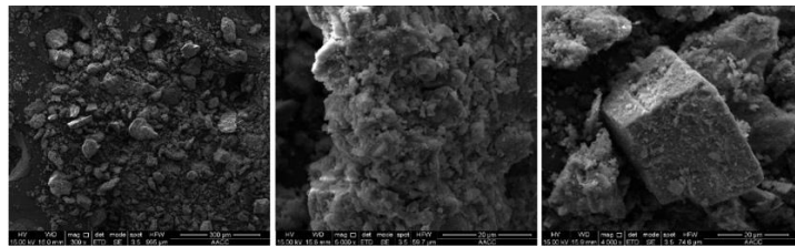
Fig. 4. SEM photos of fly ash
