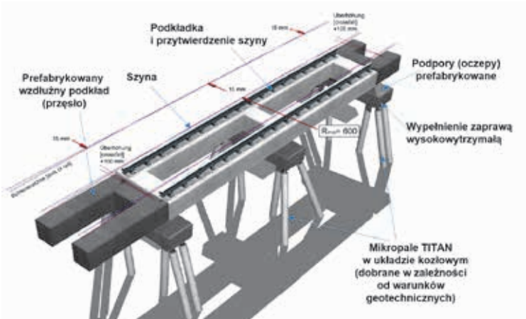
Ryc. 7. Schemat konstrukcji nawierzchni bezpodсыpkowej systemu NFF, za: [4]
