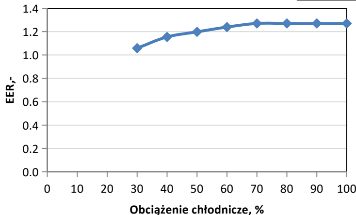
Rys. 7. Współczynnik EER dla absorpcyjnego urządzenia jednostopniowego w funkcji obciążenia [11]
