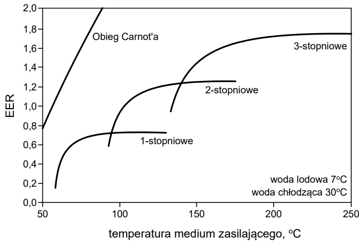
Rys. 6. Współczynnik EER urządzeń adsorpcyjnych w funkcji temperatury medium zasilającego [1]
