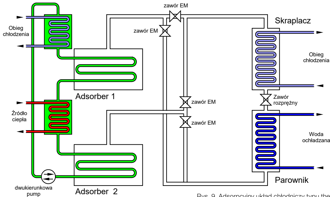
Rys. 9. Adsorpcyjny układ chłodniczy typu thermal wave
