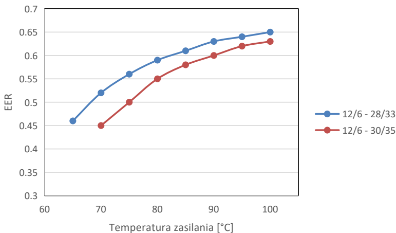
Rys. 10. EER dla urządzeń adsorpcyjnych [13]
