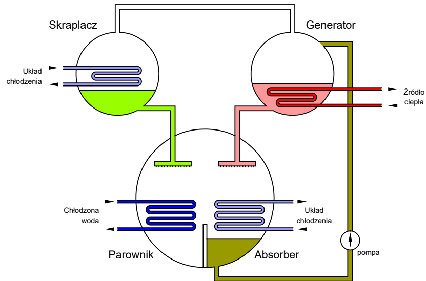
Rys. 5. Jednostopniowy układ absorpcyjny
