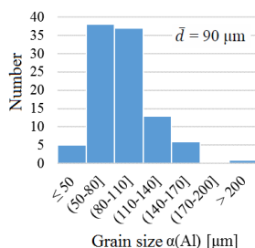
Fig. 27. Average grain size - 0,2 % AlTi5B1
