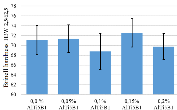
Fig. 29. Brinell hardness HBW
