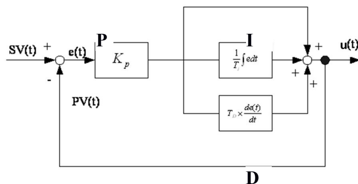
Rys. 10. Schemat blokowy regulator PID; K_p – współczynnik wzmocnienia (proporcjonalności), T_i – czas zdwojenia (całkowania), T_d – czas wyprzedzenia (różniczkowania), e(t) – odchyłka regulacji ( e(t) = SV(t) - PV(t) ), SV(t) – wartość zadana, PV(t) – wartość procesowa (mierzona) [5]
