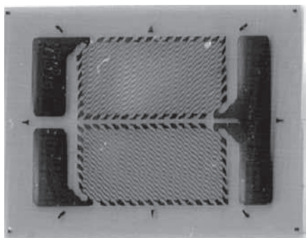
Rys. 3. Przykładowy tensometr używany do pomiaru momentu Fig. 3. Example of a strain gauge used to measure the torque
