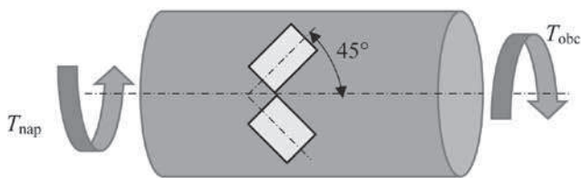
Rys. 2. Zasada pomiaru momentu skręcającego Fig. 2. Principle of torque measurements
