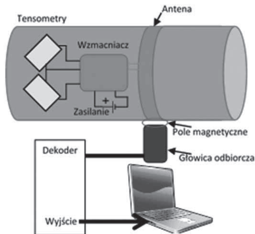
Rys. 4. Układ pomiarowy momentu obciążenia zastosowany w KGHM O/ZWR Fig. 4. Measuring system of torque applied at KGHM O/ZWR
