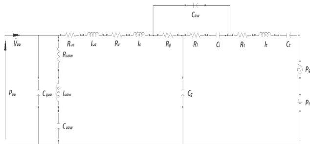
Rys. 1. 16-elementowy model układu oddechowego opisany w pracy [8] Fig. 1. 16-coefficient model of the respiratory system described in [8]
