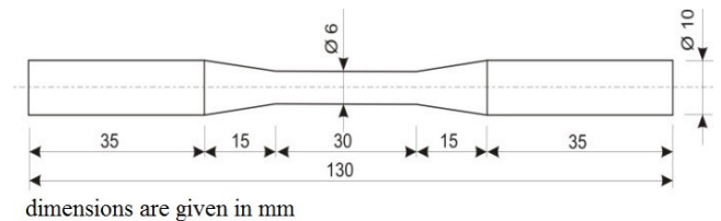
Fig. 1. Test bar 6x30 [8]
