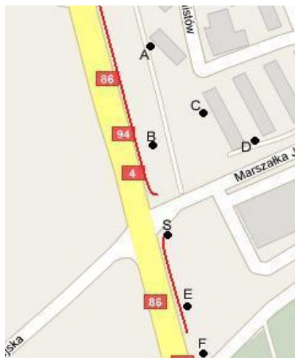
Rys. 1. Rozmieszczenie punktów pomiarowych oraz ekranów akustycznych
