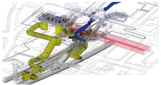
Rys. 6. Widok modelu 3D modernizacji stacji Bond Street; istniejące tunele w przezroczystych kolorach, nowe tunele w kolorze żółtym (London Underground) i niebieskim (Crossrail link) [8]
