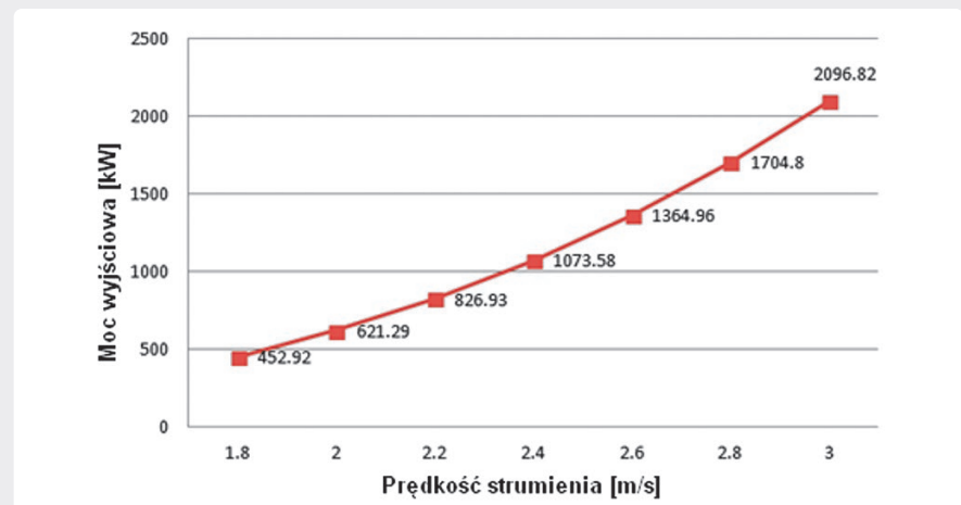
Rys. 3. Charakterystyka mocy wyjściowej turbiny w zależności od prędkości strumienia
