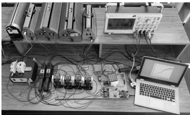
Rys. 5. Widok stanowiska laboratoryjnego
