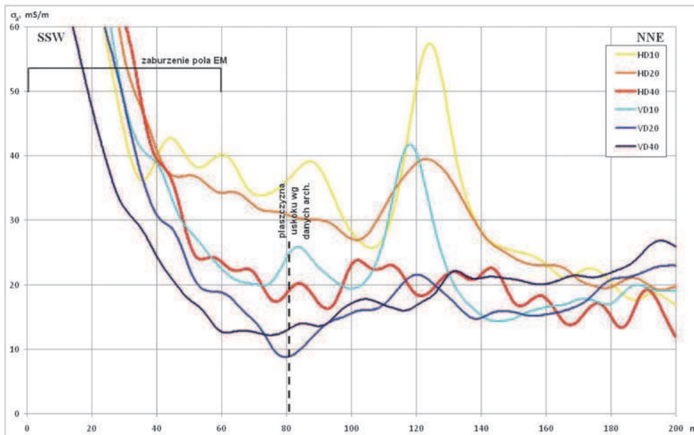
Fig. 4. Wyniki pomiarów konduktometrycznych w rejonie uskoku arkona w Katowicach Fig. 4. Results of conductivity measurements in the area of Arkona Fault in Katowice
