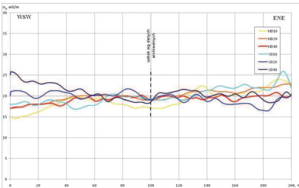
Rys. 5. Wyniki pomiarów konduktometrycznych w rejonie uskoku jakub w Katowicach Fig. 5. Results of conductivity measurements in the area of Jakub Fault in Katowice
