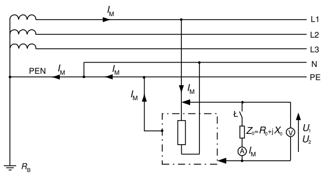
Rys. 4. Pomiar impedancji pętli zwarciowej w układzie TN
