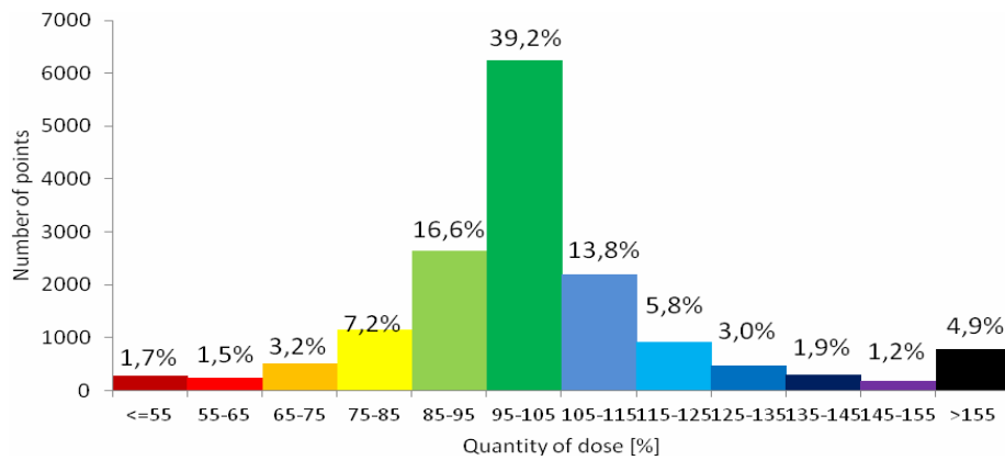
Fig. 5. The histogram of the dose of spray during crossing on the outskirts of the field in the technological paths Rys. 5. Histogram dawki oprysku podczas przejazdu po obrzeżach pola w ścieżkach technologicznych
