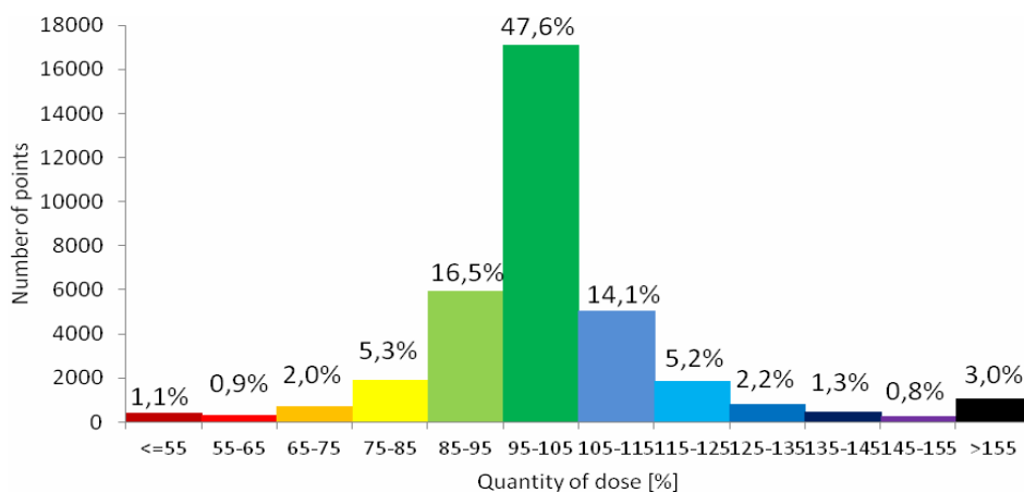
Fig. 5. The histogram of the dose of spray during crossing on the outskirts of the field in the technological paths Rys. 5. Histogram dawki oprysku podczas przejazdu po obrzeżach pola w ścieżkach technologicznych
