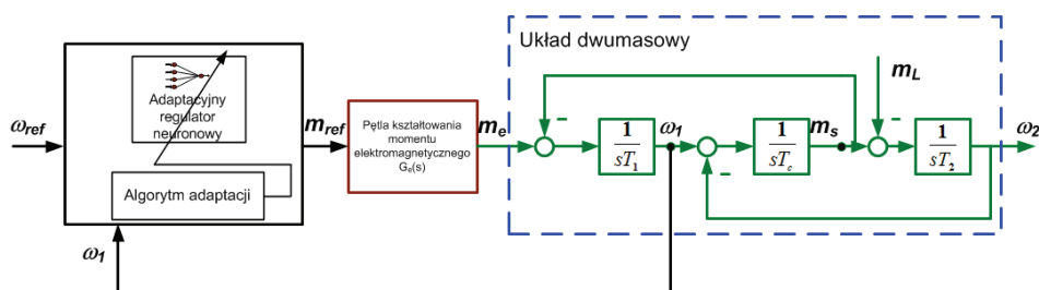
Rys. 1. Schemat blokowy uproszczonego modelu układu napędowego z dynamicznym sterowaniem momentu elektromagnetycznego
