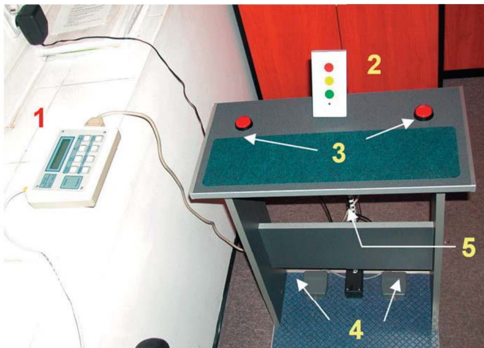
Rys. 1. Miernik czasu reakcji MCR - 2001E, 1 - jednostka centralna MCR - 2001 E - mikroprocesorowy miernik czasu reakcji, 2 - semafor (sygnalizator - wyzwalacz bodźców świetlnych i bodźca dźwiękowego), 3 - manipulatory „ręczne”, 4 - manipulatory „nożne”, 5 - układ przyłączeniowy
