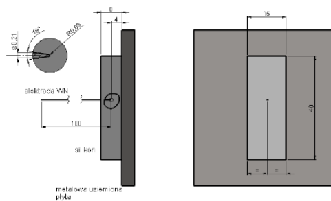
b) układ generujący wyladowania typu korona
