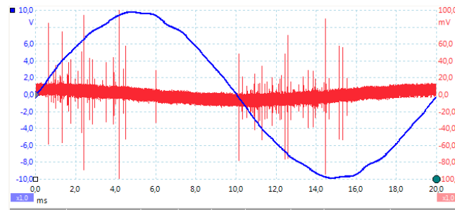
c) wartość skuteczna napięcia probierczego 6,8 kV, czas pomiaru 20 ms
