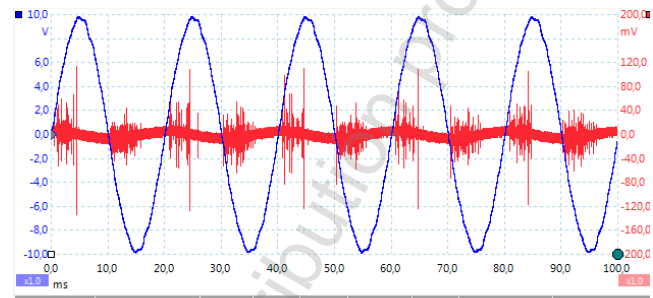
d) wartość skuteczna napięcia probierczego 6,8 kV, czas pomiaru 100 ms
