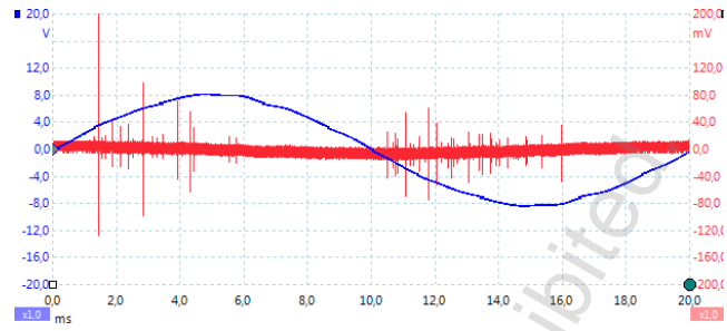
b) wartość skuteczna napięcia probierczego 5,7 kV, czas pomiaru 20 ms
