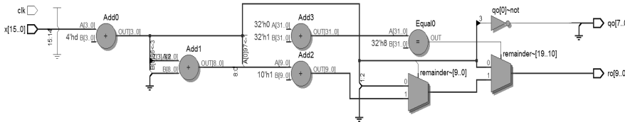
Rys. 7. Układowa implementacja algorytmu metody nieodtworzącej obliczania PK na poziomie RTL – struktura z ALU
