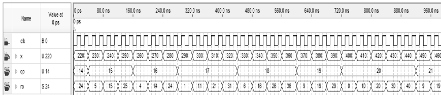
Rys. 8. Wynik symulacji układowej implementacji algorytmu metody nieodtworzącej obliczania PK ( x – liczba podpierwiastkowa, qp – wartość całkowita pierwiastka, ro – wartość całkowita reszty)
