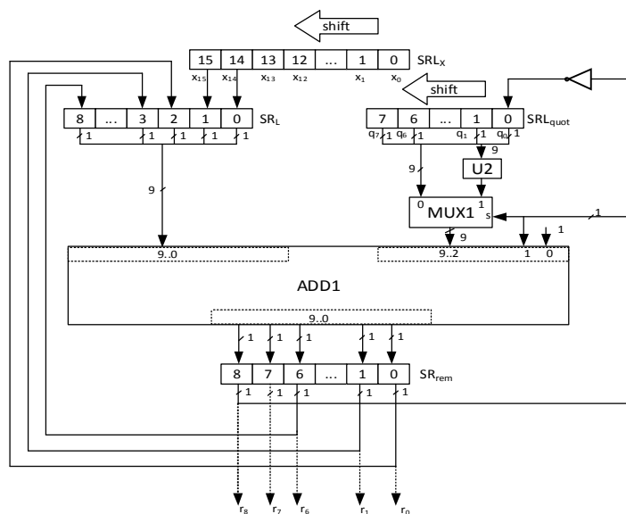
Rys. 4. Schemat blokowy implementacji układowej algorytmu metody nieodtworzającej obliczania PK dla zakresu n = 16
