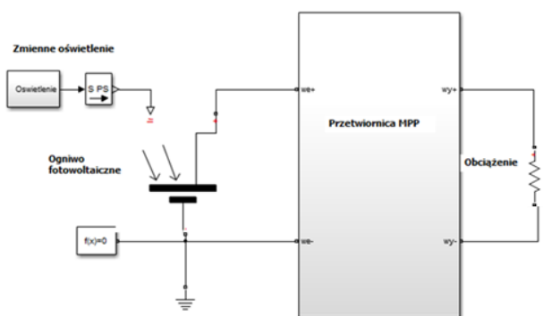
Rys. 2. Schemat badanego układu
