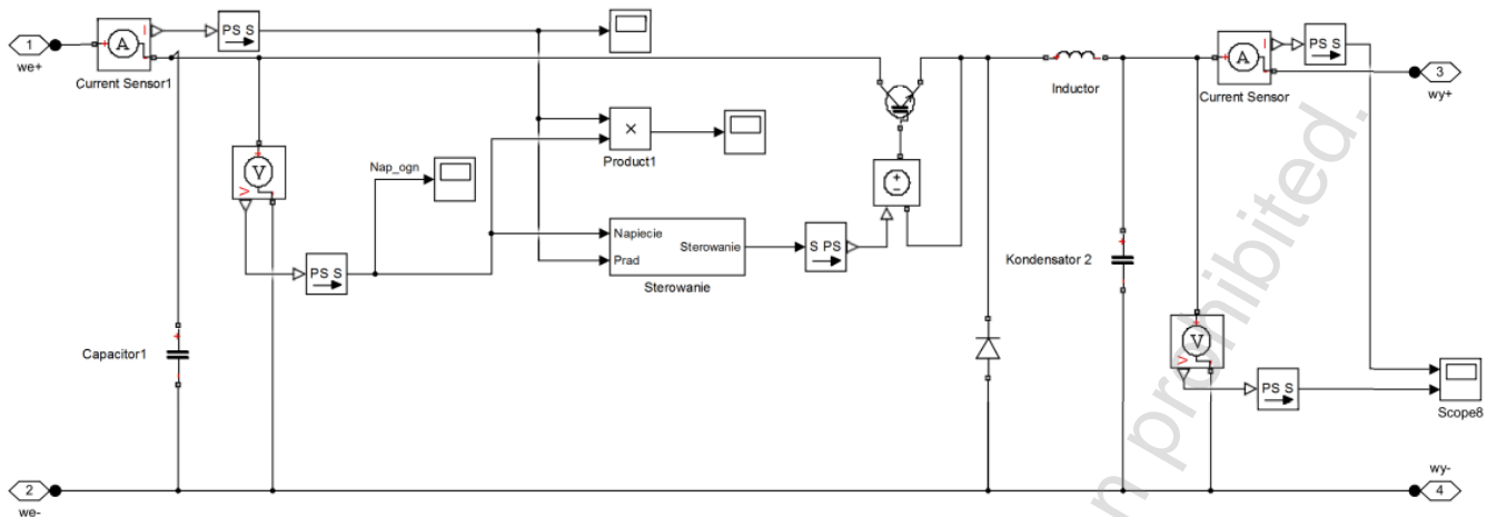
Rys. 3. Schemat przetwornicy MPP
