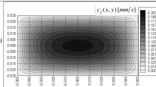
Rys. 5c. Rozkład prędkości przepływu w przewodzie prostoosiowym o przekroju prostokątnym A/B=2 , Re=50 . Wykres warstwiczny pola prędkości
