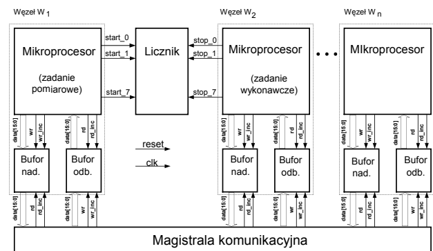
Rys. 1. Model strukturalny RSPS
