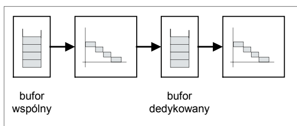
Rys. 3. Struktura węzła wykonawczego z buforem dedykowanym Fig. 3. Structure of executive node with dedicated buffer
