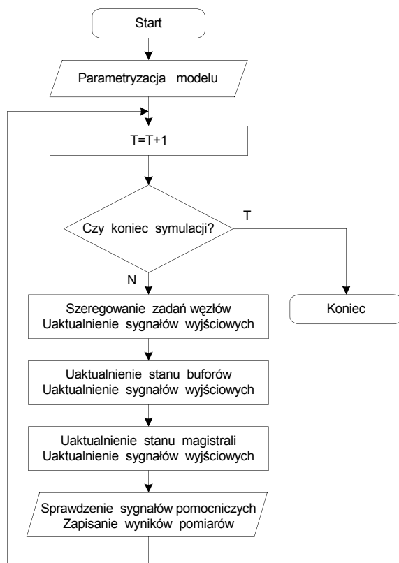
Rys. 2. Algorytm pracy programu realizującego model RSPS Fig. 2. Algorithm of a simulation model program
