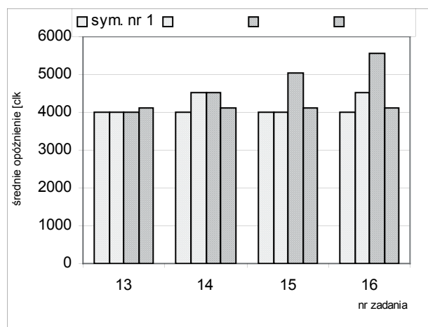
Rys. 7. Średnie opóźnienia w transmisji danych dla przypadku: 1, 7, 9, 11 dla zadań systemu o najdłuższym okresie występowania
