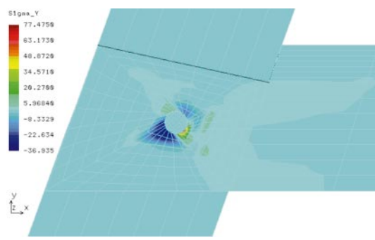
Model III – Naprężenia normalne \sigma_y – ściskanie jętki
