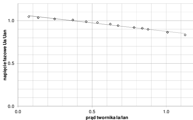
Charakterystyka zewnętrzna U_a=f(I_a)
