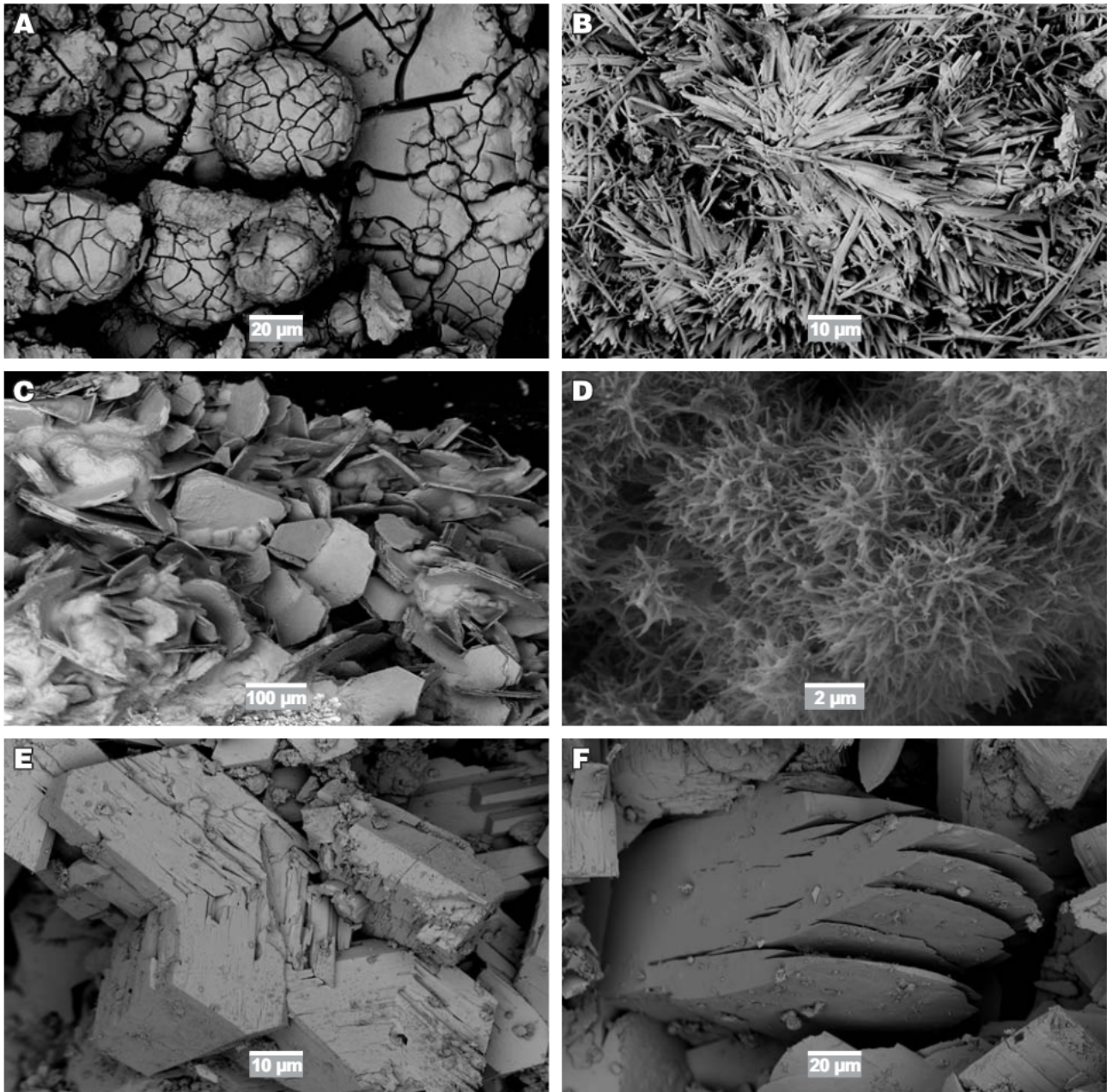
Ryc. 2. A – powłoka skorodytu na arsenopirycie; B – igielkowe kryształy zýkaitu; C – tabliczkowe kryształy goethytu; D – jeżykowe skupienia schwertmannitu; E – bliźniak kryształów langitu; F – tabliczkowe kryształy brochantytu
