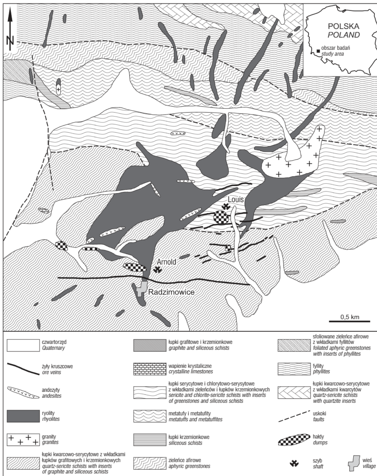
Ryc. 1. Mapa geologiczna obszaru złoża w Radzimowicach według Mikulskiego (2005), zmienione Fig. 1. Geological map of the area of the Radzimowice deposit after Mikulski (2005), modified
