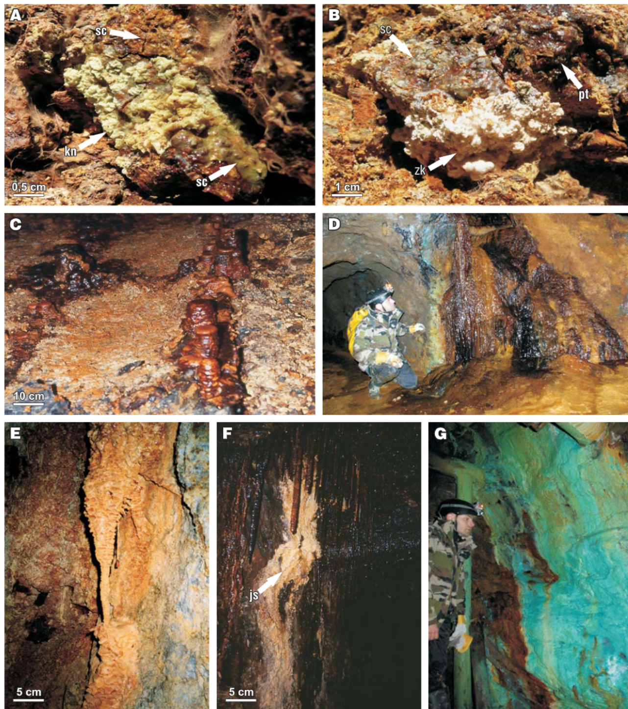
Ryc. 3. A – zielonożółte naskorupienia kaňkitu (kn) współwystępującego ze skorodytem (sc); B – kuliste skupienia białego zýkaite (zk) współwystępującego ze skorodytem (sc) i pitticytem (pt); C – stalagmity pitticytu; D – brunatne nacieki schwertmannitu; E – rdzawe nacieki ferrihydrytu; F – żółte nagromadzenia hydroniojarosytu (js) stowarzyszone z brunatnymi stalaktytami tlenowodorotlenków żelaza; G – zasadowe siarczany miedzi na ścianach starego chodnika górniczego
