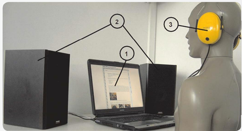
Rys. 2. Widok systemu do nauki prawidłowego użytkowania środków ochrony indywidualnej słuchu: 1 – komputer z oprogramowaniem, 2 – źródłami sygnału testowego, 3 – szkoleniowiec ochronniki słuchu
