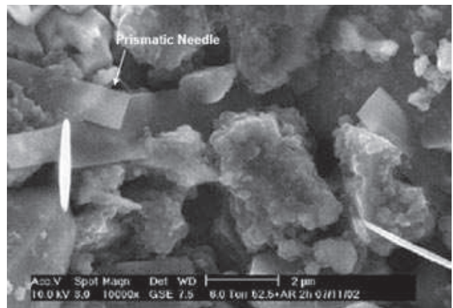
Rys. 2. Fotografia SEM zaczynu cementowego modyfikowanego dodatkiem 3% organicznego reduktora skurczu SRA [3]
