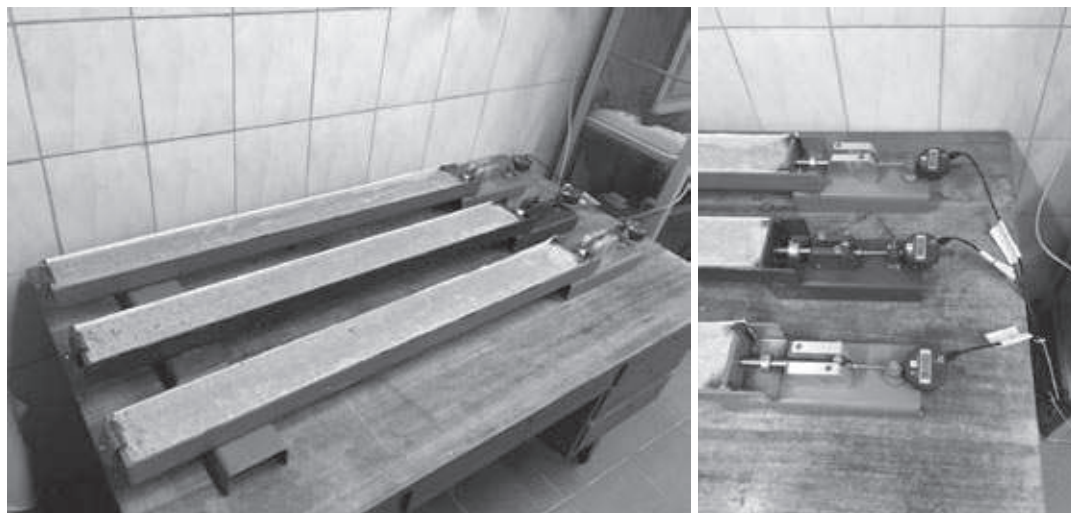
Rys. 3. Rynny skurczowe z zamontowanymi czujnikami przemieszczeń rejestrującymi zmiany długości próbek
