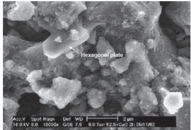
Rys. 1. Fotografia SEM zaczynu cementowego modyfikowanego 3% dodatkiem domieszki ekspansywnej na bazie CaO – widoczne hexagonalne kryształy portlandytu [3]
