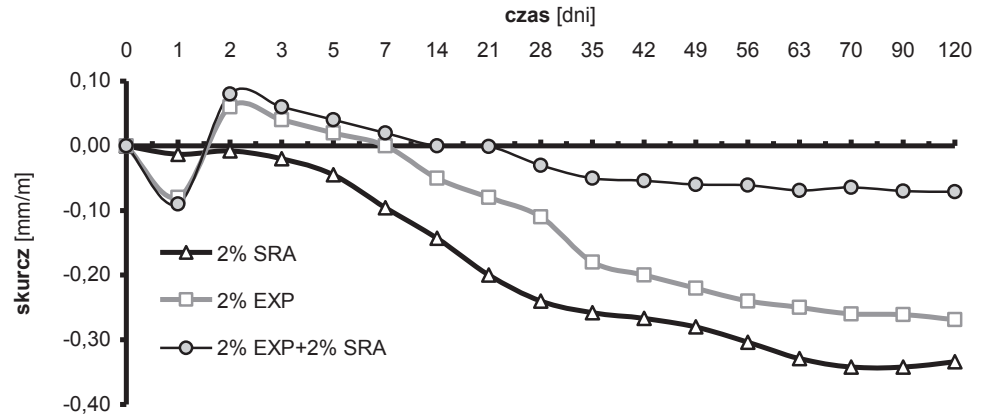
Rys. 6. Przebieg skurczu zapraw modyfikowanych domieszką MAPEPURE SRA (2% m.c.) i domieszką ekspansywną EXPANCRETE (2% m.c.)
