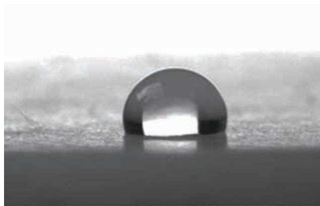
Fot. 2. Kształt kropli na powierzchni hydrofobowej (płytki teflonowej, kąt zwilżania między 90^\circ a 120^\circ )
